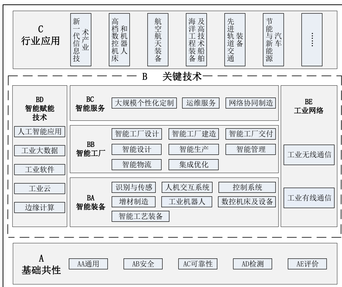
图 2 智能制造标准体系结构图
